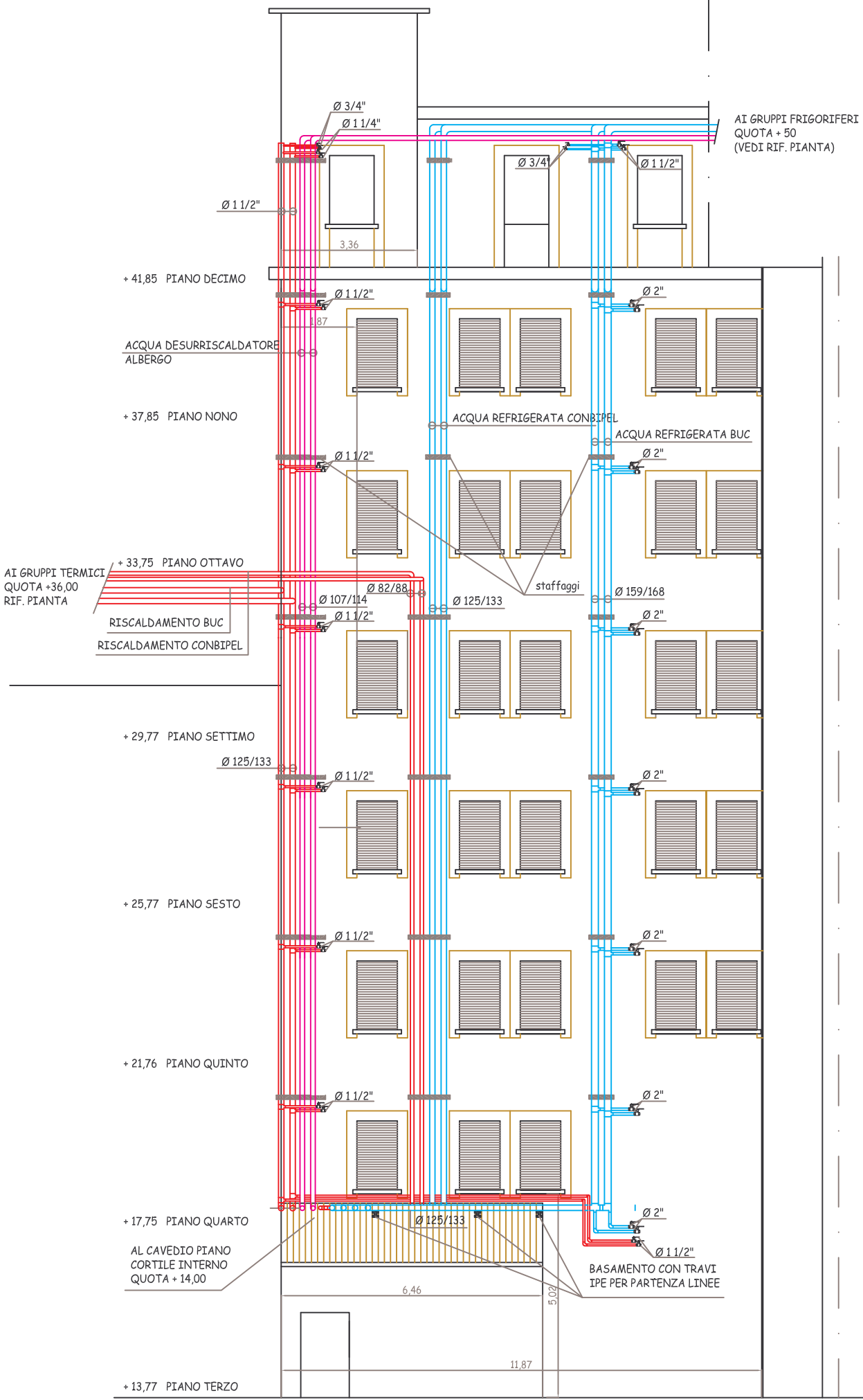
VISTA PASSAGGIO TUBAZIONI IMPIANTI MECCANICI PROSPETTO INTERNO LATO CORTILE ALBERGO
